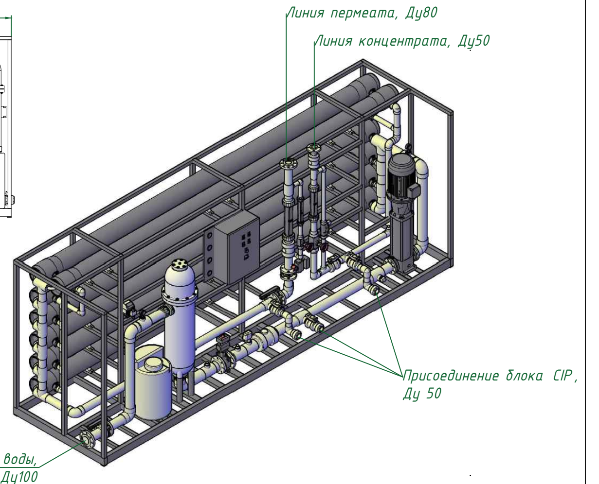
Изометрия
