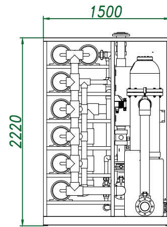
Вид слева
