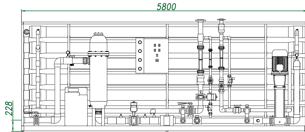
Вид спереди
